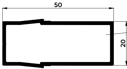
01253 LAMA 50X20
