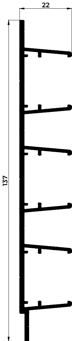
01254 SOPORTE LAMA
