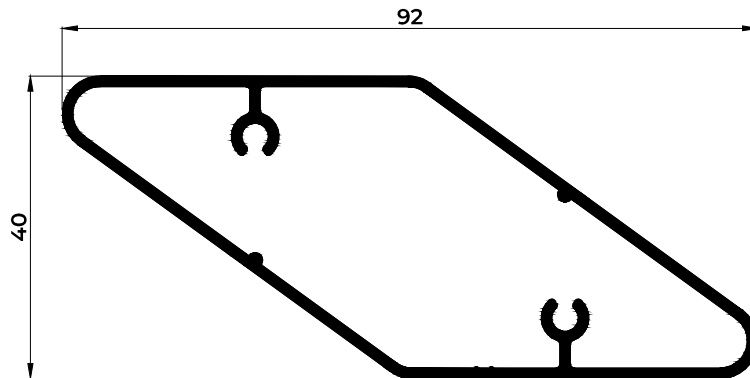
01357 LAMA DE 92 PORTATORNILLOS
