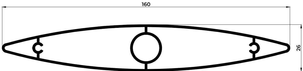
01251 LAMA REGULABLE DE 160 (ACCESORIO DISPONIBLE)
