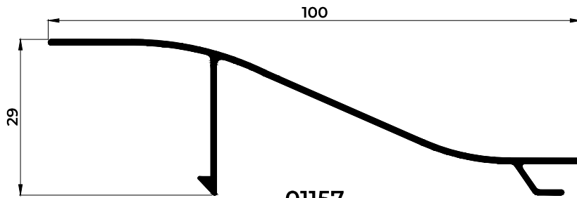
LAMA FIJA DE 100 CURVA
