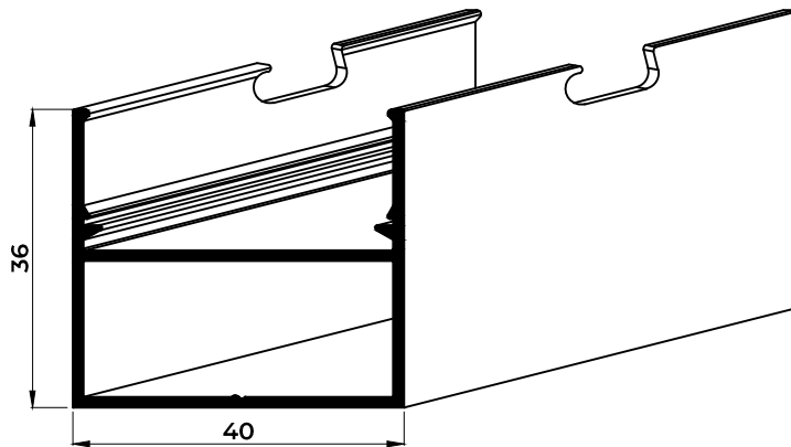
MARCO LISO VENTANA TROQUELADO
