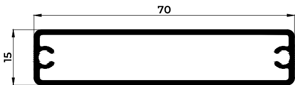
01258 TUBO 70X15 PORTATORNILLOS
