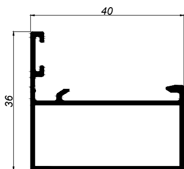
40030 MARCO LISO
