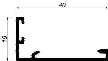
40023 BATIENTE MARCO
