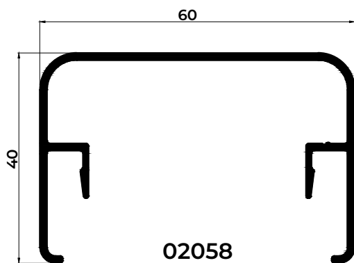
PASAMANOS CUADRADO DE 60x40
