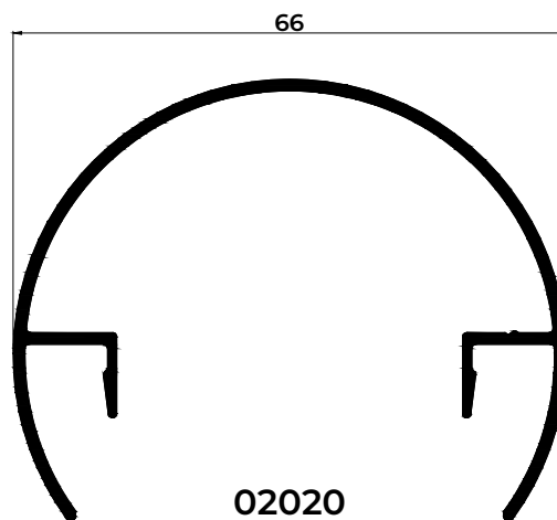
PASAMANOS REDONDO DE 66
