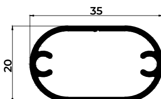
02125 OVALADO DE 35x20
