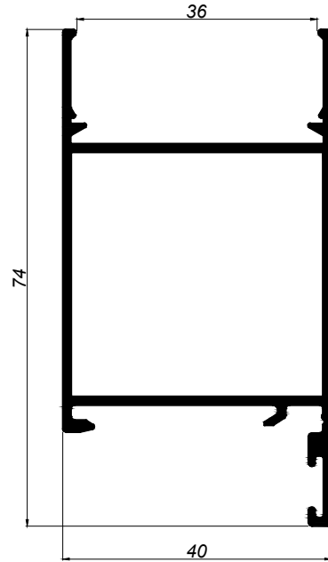
01029 HOJA PUERTA
