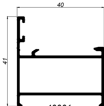
40001 MARCO VENTANA
