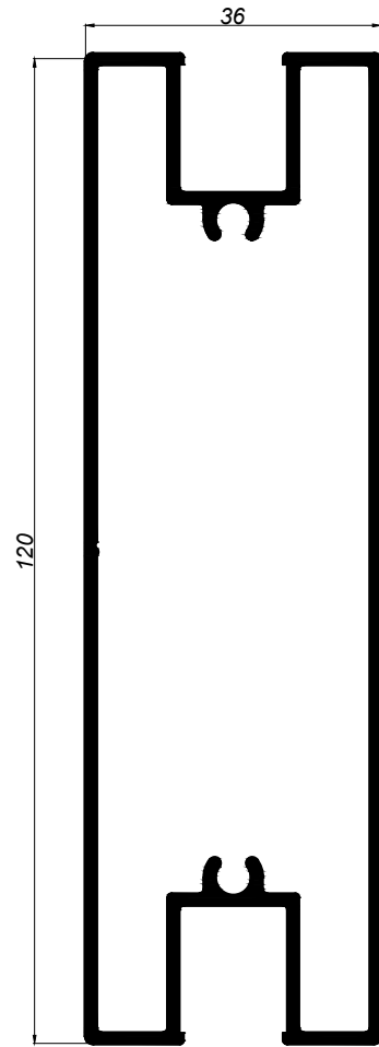
01110 ZOCALO DIVISOR DE 120
