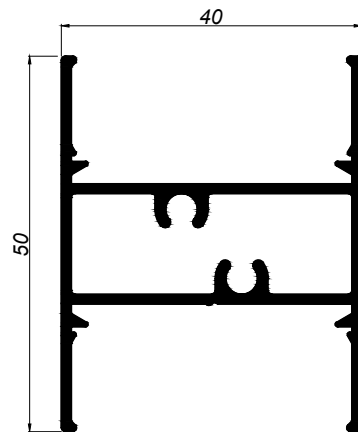
01013 PILASTRA PORTATORNILLOS
