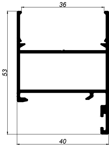
01006 HOJA VENTANA
