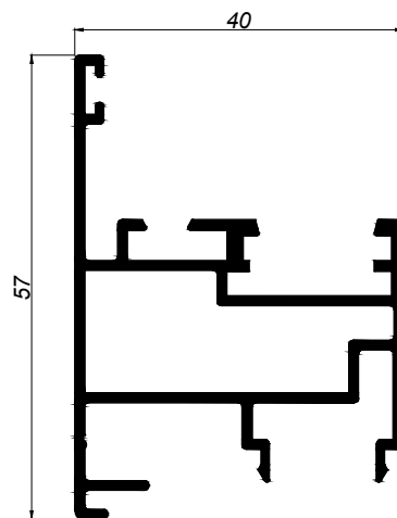
47105 INVERSOR RECTO
