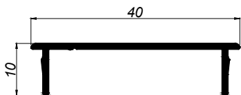
01030 TAPETA MALLORQUINA
