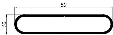
01008 LAMA FIJA
