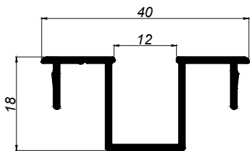
01102 PERFIL OMEGA
