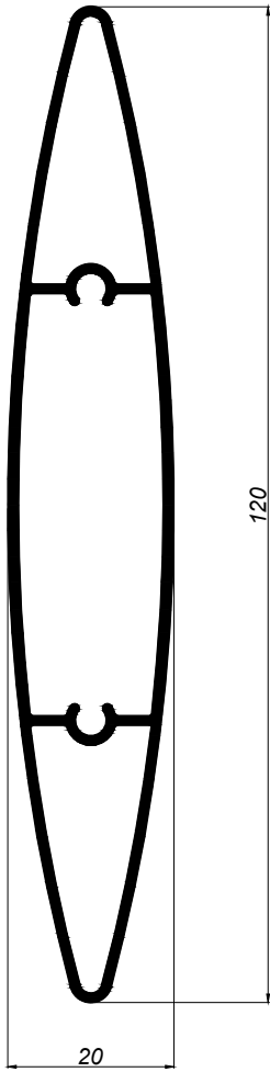
01252 LAMA OVAL DE 120
