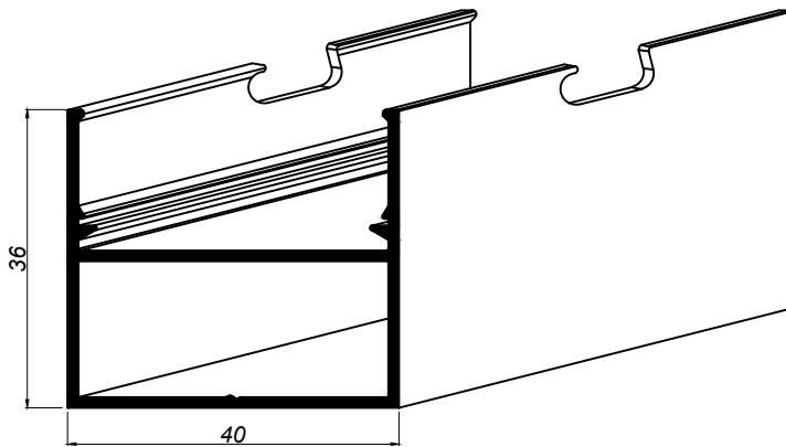
01053 MARCO LISO VENTANA TROQUELADO
