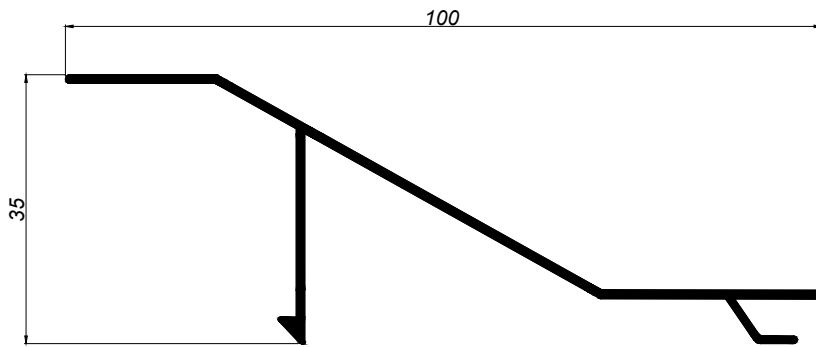
01446 LAMA FIJA DE 100 RECTA
