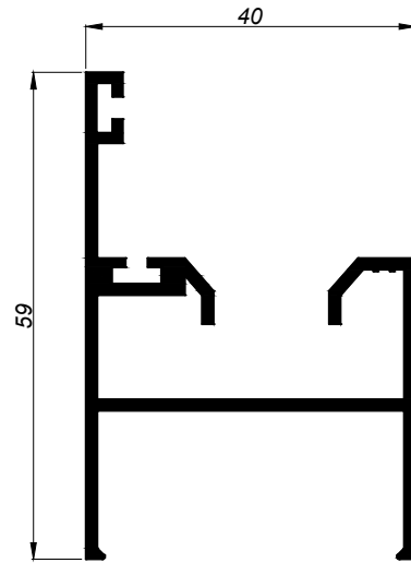
41003 MARCO INFERIOR
