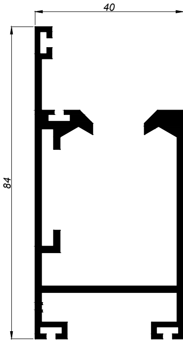
41000 MARCO SUPERIOR
