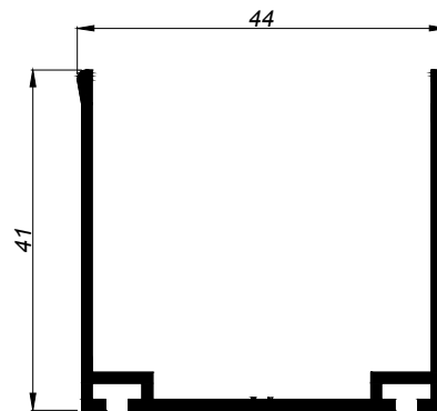
41005 PERFIL COMPENSADOR
