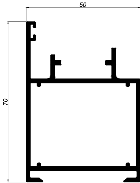
50050 MARCO PUERTA
