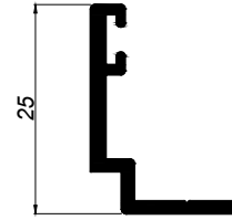
50055 BATIENTE FIJO
