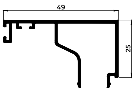
32016 TAPA MONOCARRIL
