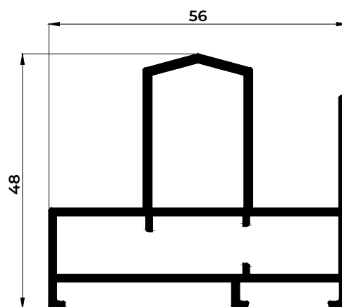
32018 MARCO ENTREMUROS
