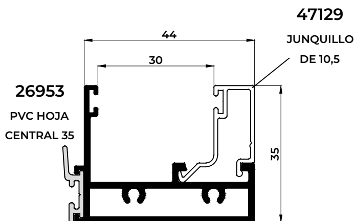
32017 CRUCE MONOCARRIL
