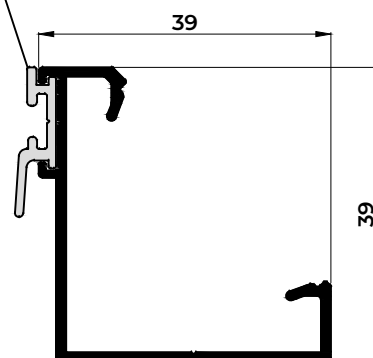
32019 CRUCE ENTREMUROS
