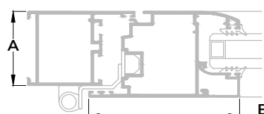
PUERTA
